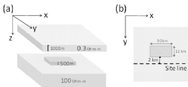
第1図 (a)フォワード計算に用いた3次元モデル。(b)モデル平面図
