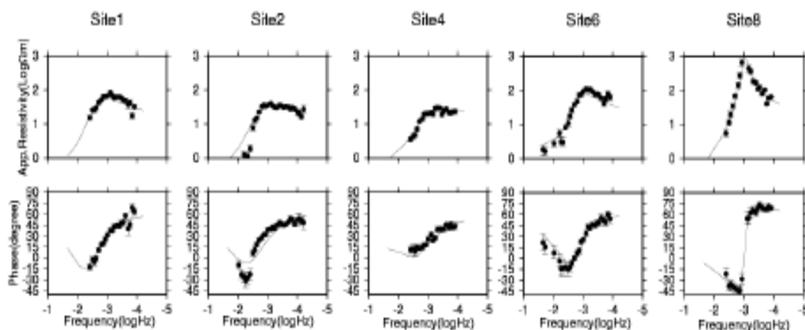
第 8 図 5 地点での TE モードの見掛け比抵抗値と位相差。
