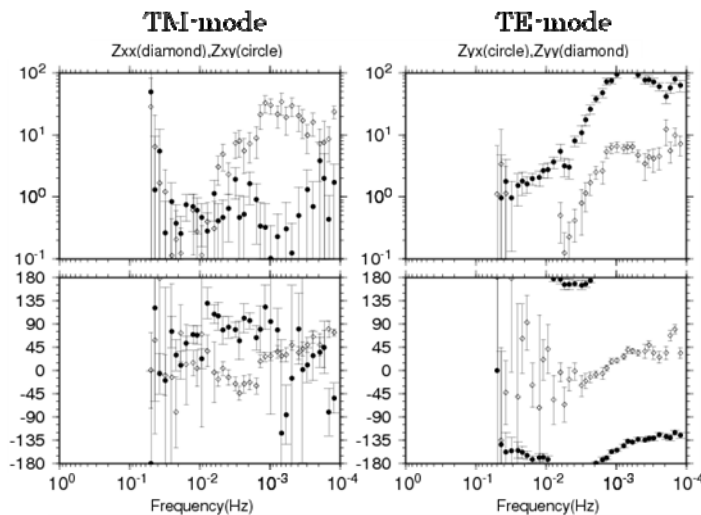
第 5 図 Site1 での MT レスポンス。黒い点は Zxy もしくは Zyx、白い点は Zxx もしくは Zyy。
